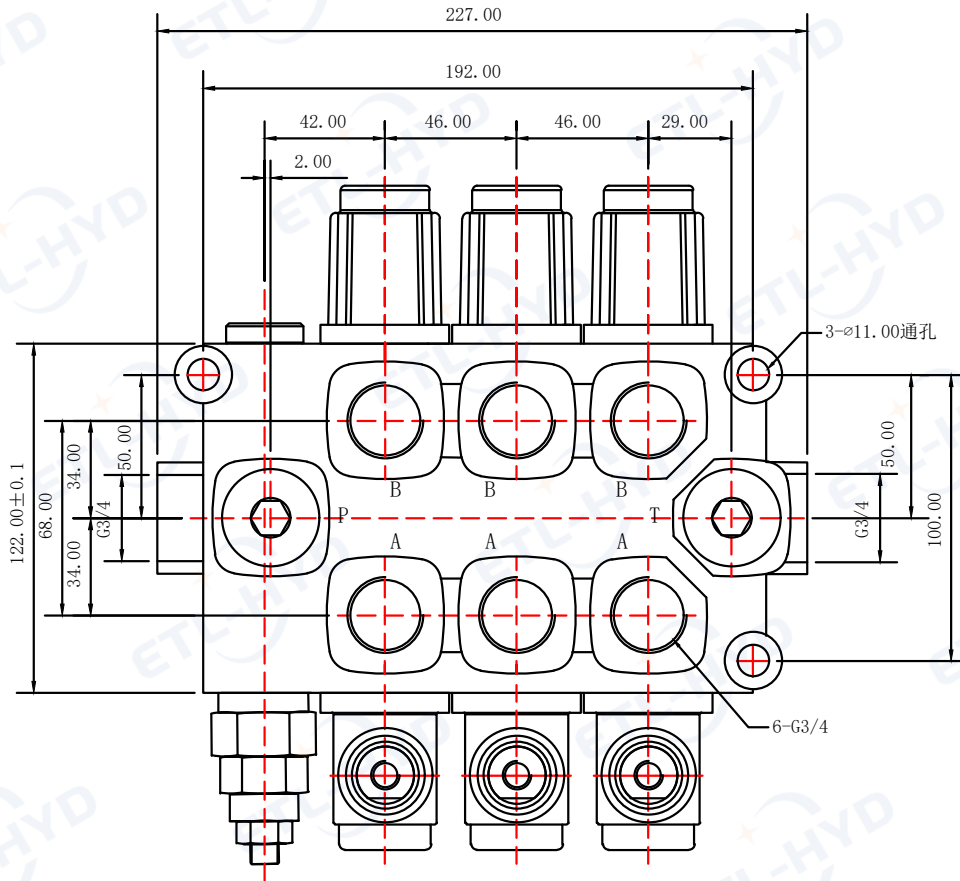
Q95 外形安装连接尺寸/MODEL Q95 DIMENSIONAL DATA
